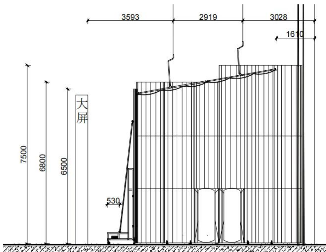
反声罩侧视图
