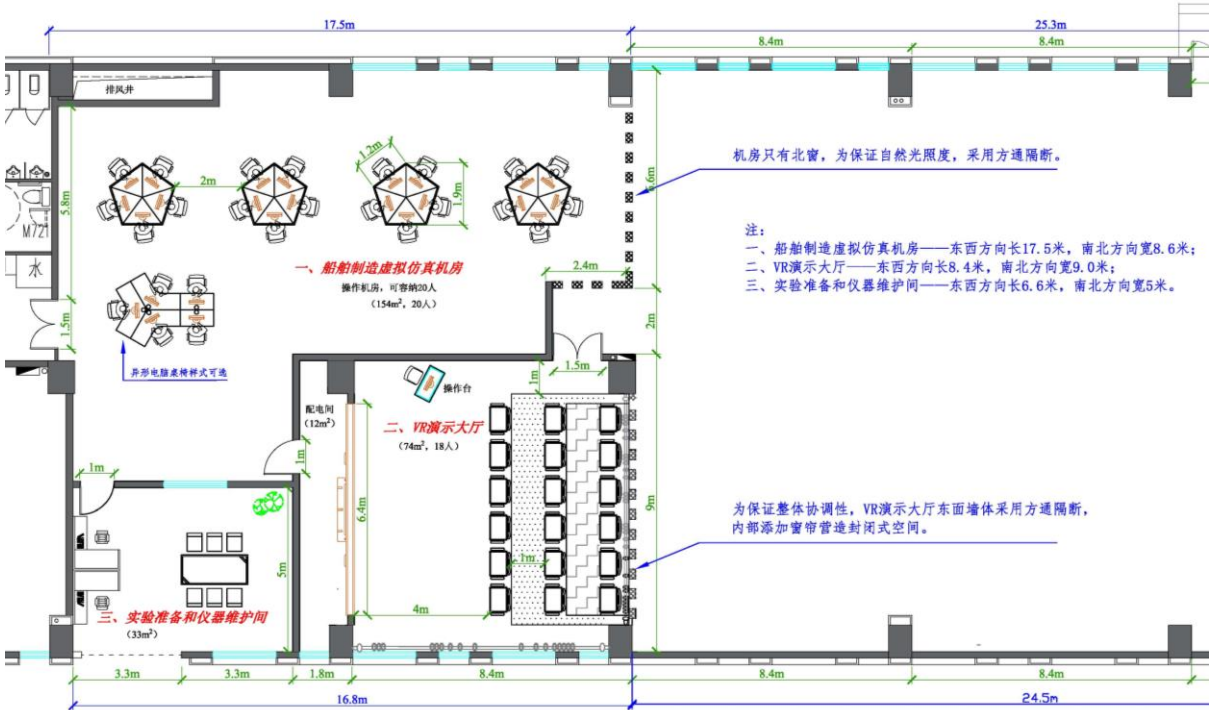
图 2 拟建设规划平面图
